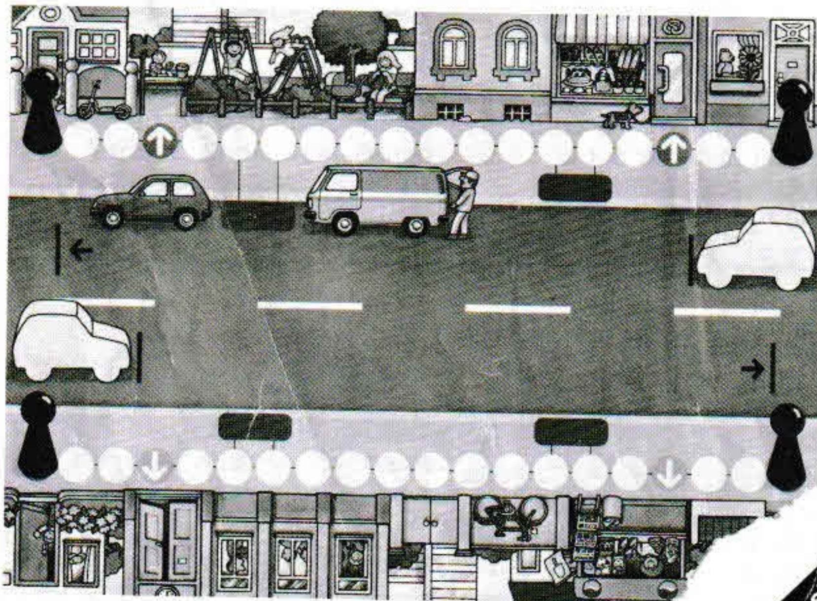
Schéma 1: position de départ. Les autos se trouvent sur les traits n le sens de la circulation.
