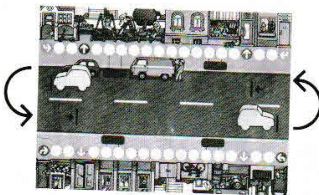
Schema 2: les autos sont mises en sens inverse.
